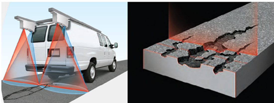
Figuur C.3 Werkingsprincipe LCMS.
