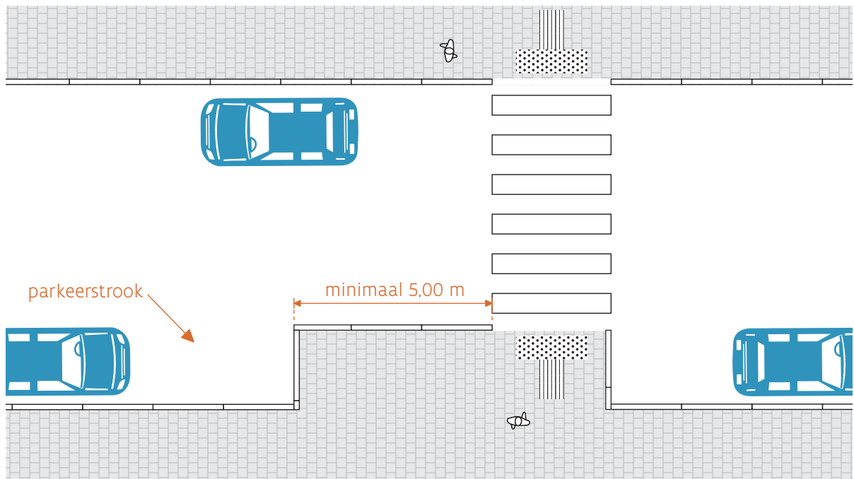
Figuur 5: Uitstulpend voetpad
